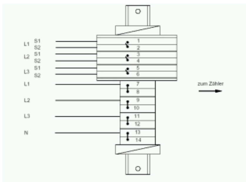
Bild 1 - Klemmenleiste für Wandleranlagen
